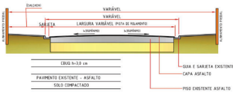
PERFIL TRANSVERSAL DAS VIAS PÚBLICAS
